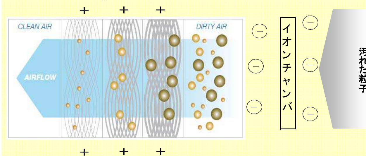
HEPASilent™テクノロジーの構造
